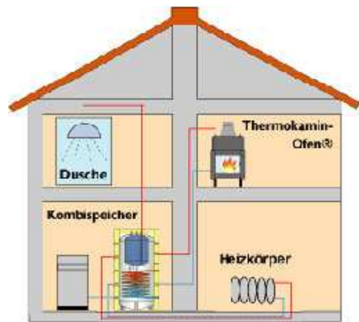
Heizen in Verbindung mit einem Öl- oder Gaskessel
