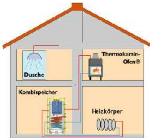
Heizen mit den Thermokamin- Ofen®
